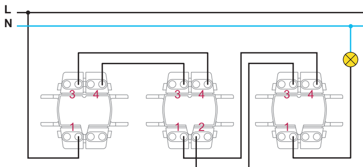
2 проходных переключателя + перекрестный переключатель
