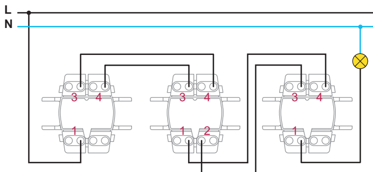
2 проходных переключателя + перекрестный переключатель с подсветкой
