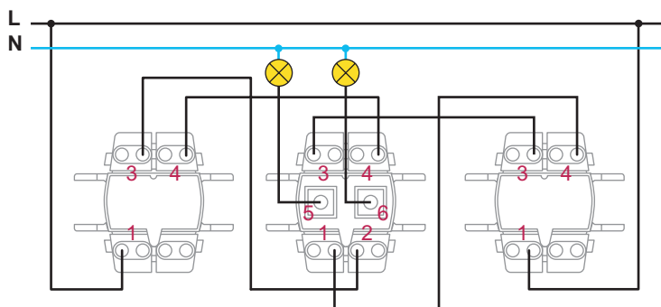
2 проходных переключателя + двухклавишный переключатель
