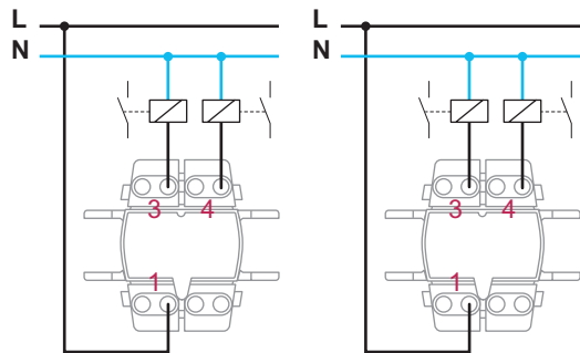
Кнопочный переключатель
